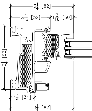
⑦ 800 SLIDER JAMB
