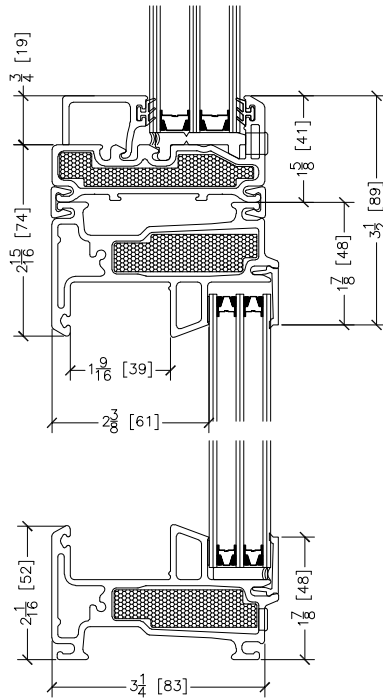
④ 800 SLIDER SILL
